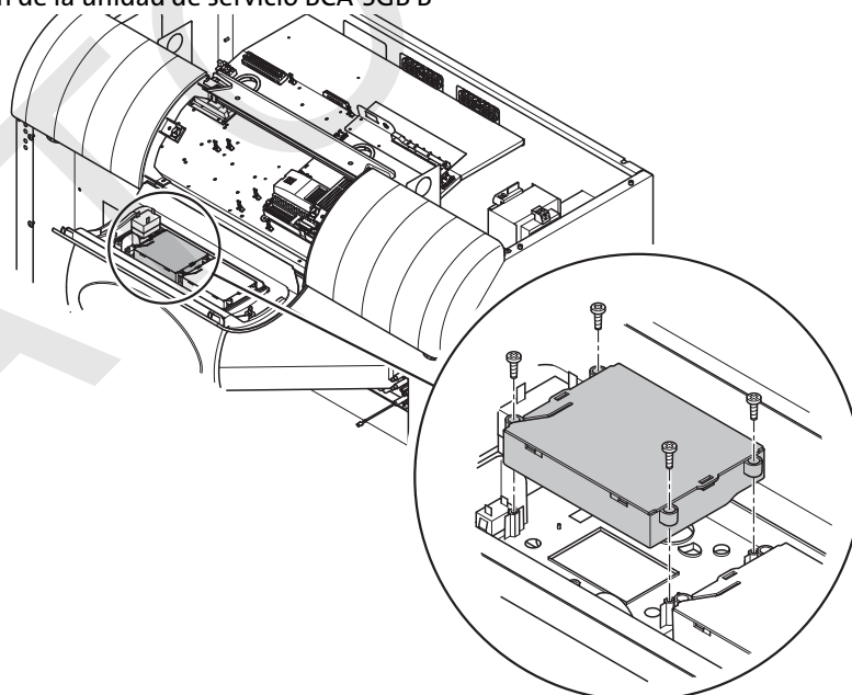
Fig. 8: Colocación de la unidad de servicio BCA-SGB B
