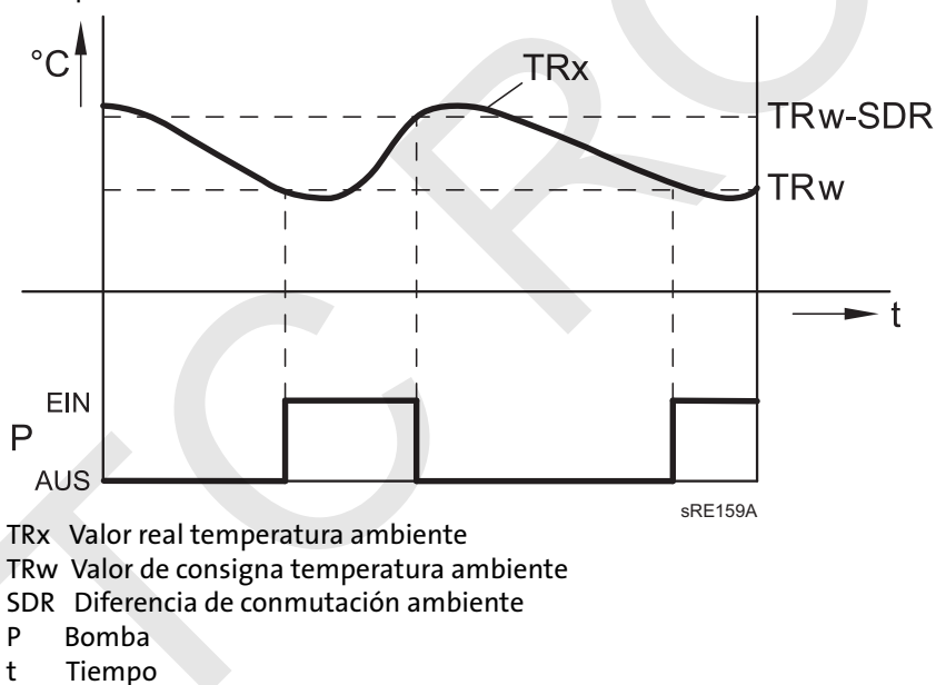
Fig. 18: Limitación temp. ambiente
