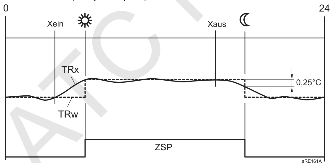
Fig. 20: Control marcha óptima y control paro óptimo
