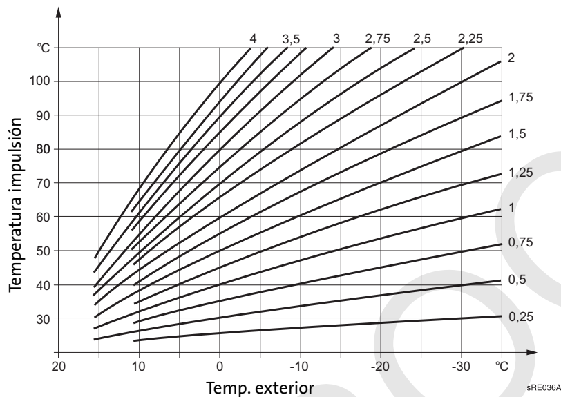
Fig. 16: Diagrama de la curva de calefacción
