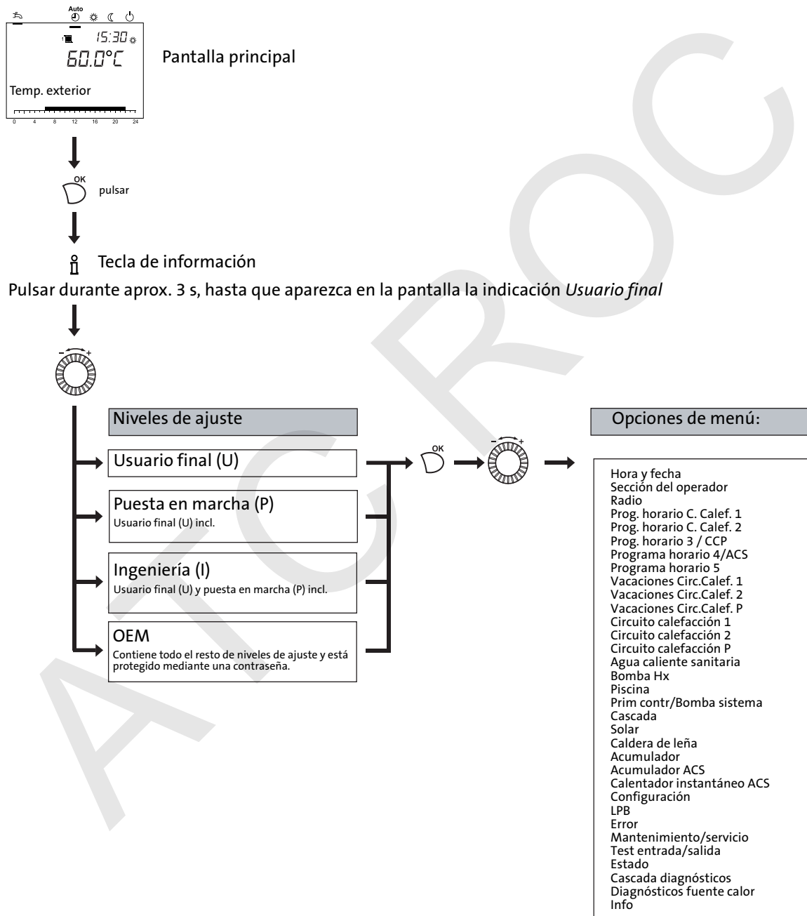
Fig. 15: Selección de los niveles de ajuste y opciones de menú
