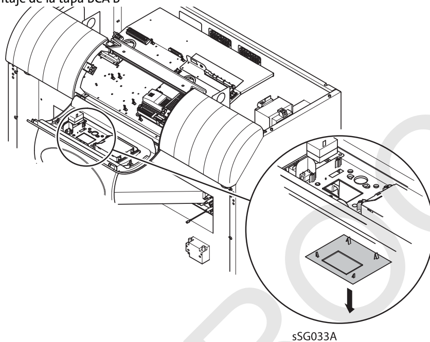
Fig. 7: Desmontaje de la tapa BCA B
