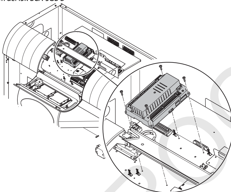
Fig. 9: Colocación del ISR BCA-SGB B
